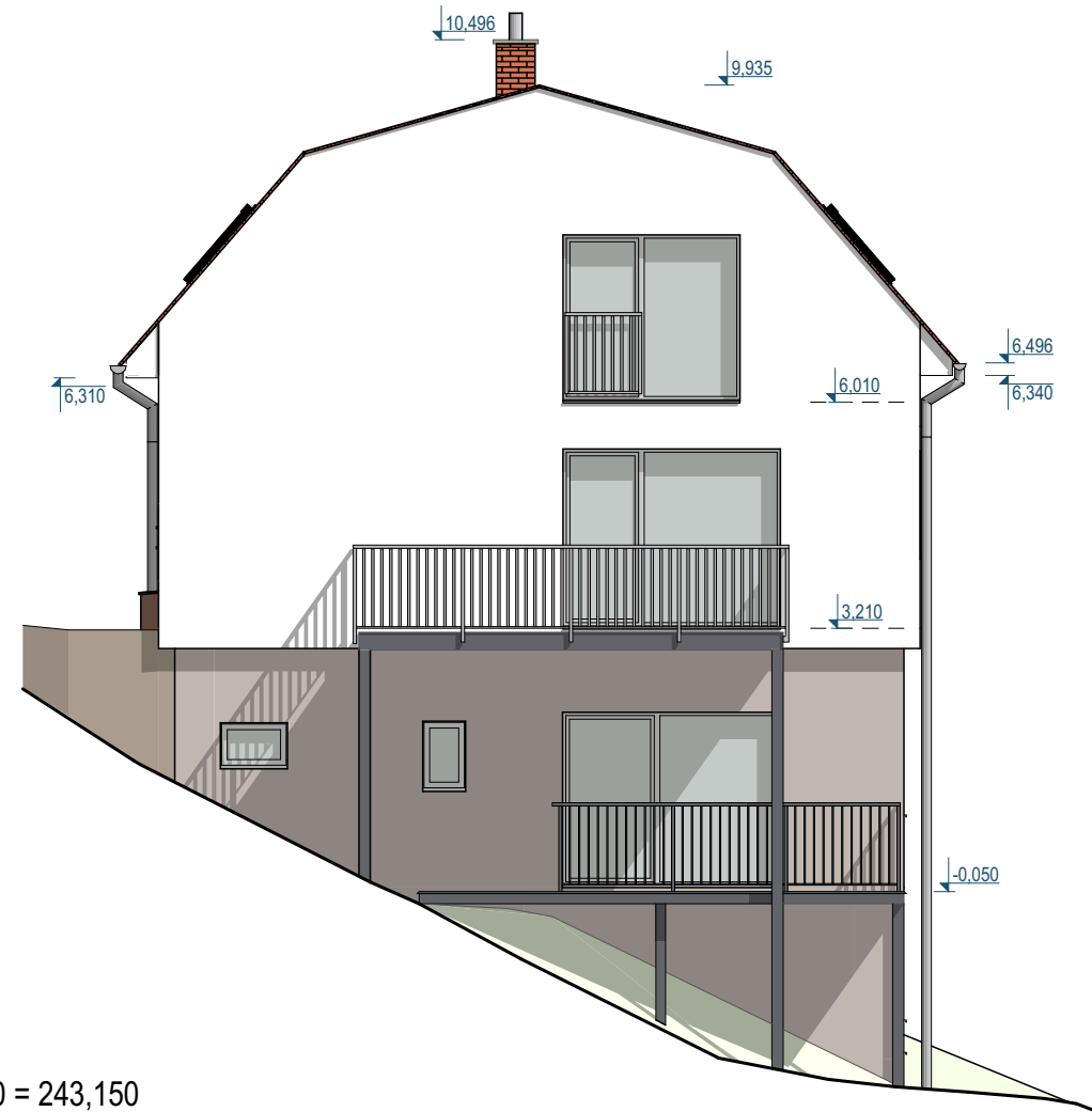
Pohled severozápadní
