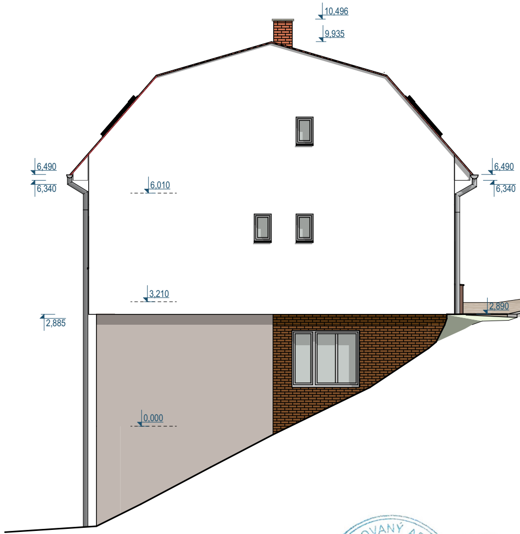
Pohled jihovýchodní
